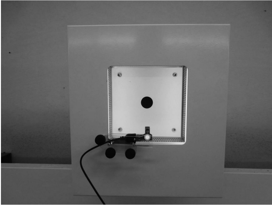
USB給電式汎用タイプの赤外線ユニットをMeyton社製の標的に搭載した例
