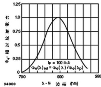
図 9-相対放射電力 対 波長
